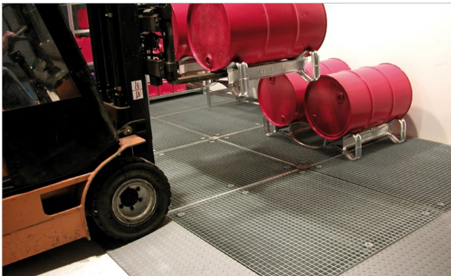
8 x BSW + 6 x AR + 1 x AE + 3 x KV + 10 x WV (Zubehör: Fasspaletten FP-2, Fassregale FR)
