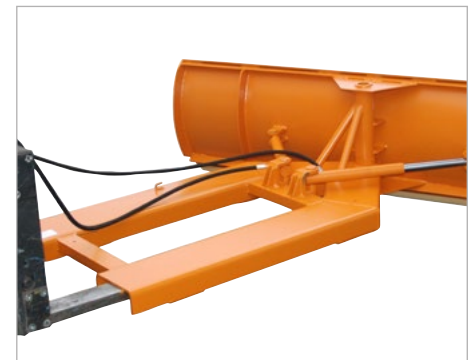
Hydraulische Schildverstellung
